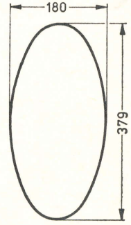
E379x180.1 Konkav
