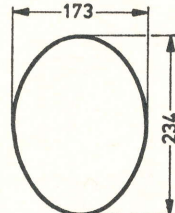
E 234 × 173.1 Konkav
