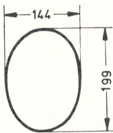
E 199 x 144.1 Konkav
