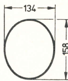
E 158 x 134.1 Konkav
