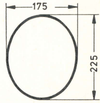
E 225x175.1 Konkav
