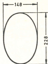
E 228 × 148.1 Konkav
