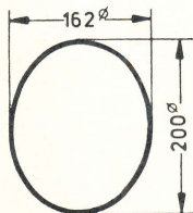
E 200 x 162.1 Konkav
