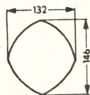
E 146 x 132 . 1 Konkav
