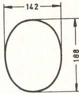
E 188 x 142 1 Konkav
