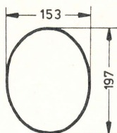
E 197 x 153.1 Konkav
