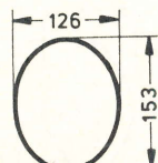
E 153 x 126.1 Konkav
