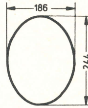
E 244 x 186.1 Konkav
