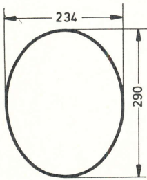
E 290 x 234.1 Konkav
