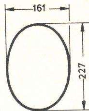
E 227 × 161.1 Konkav
