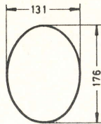
E 176 x 131.1 Konkav
